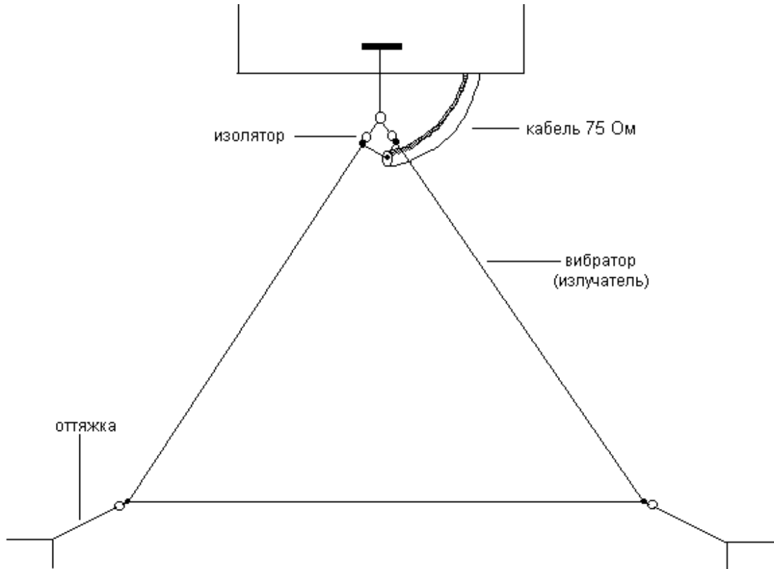
Рис.2.12. Антенна «треугольник»
